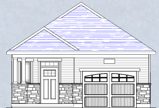
ELEVATION B
